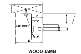
WOOD JAMB
